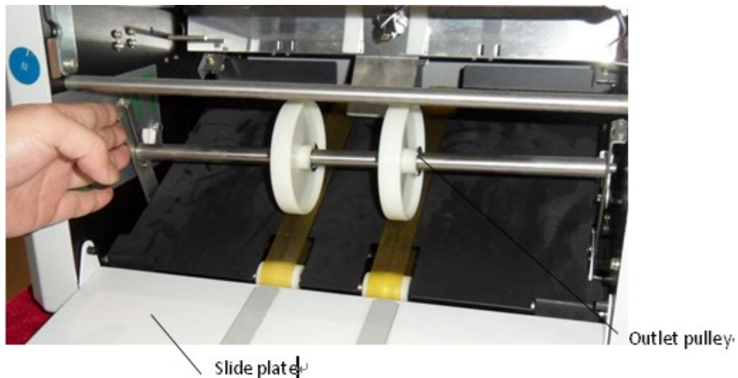
Fig.10 Outlet pulley
